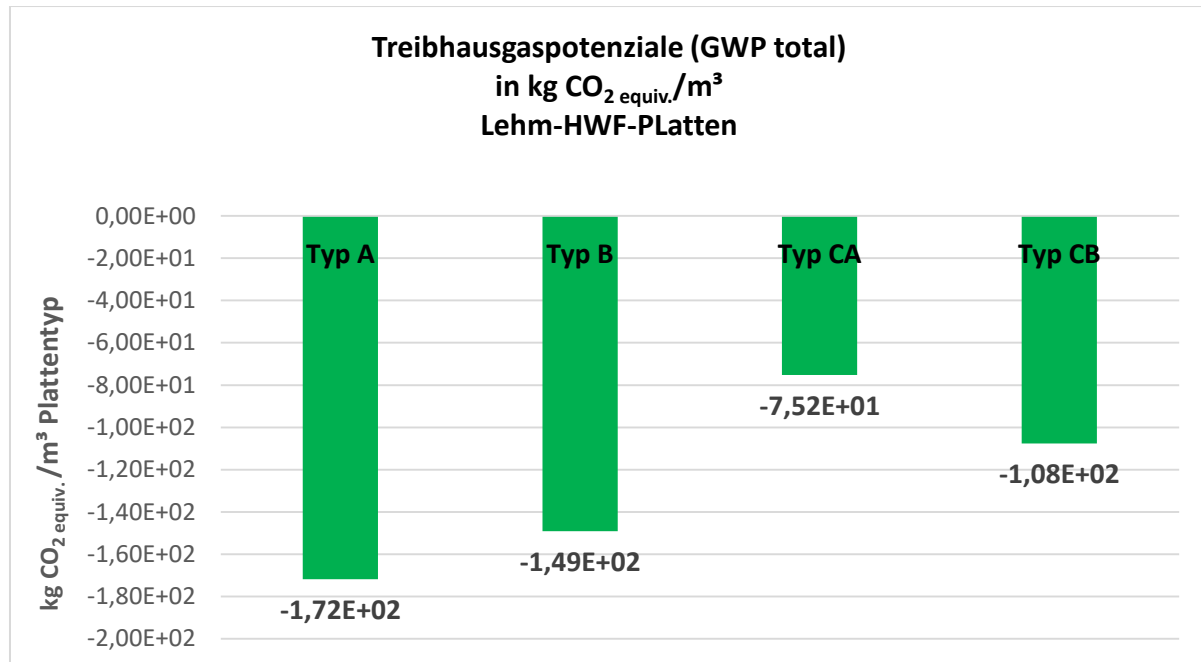
Abb. C.3 Treibhausgaspotenziale GWP pro \text{m}^3
